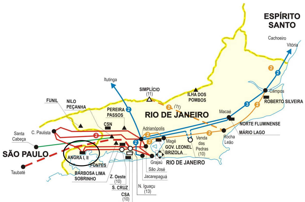
Figura 3-1: Diagrama Eletrogeográfico
